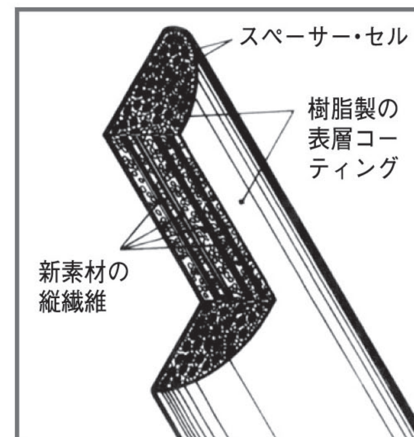
ファイブラセルの断面図
